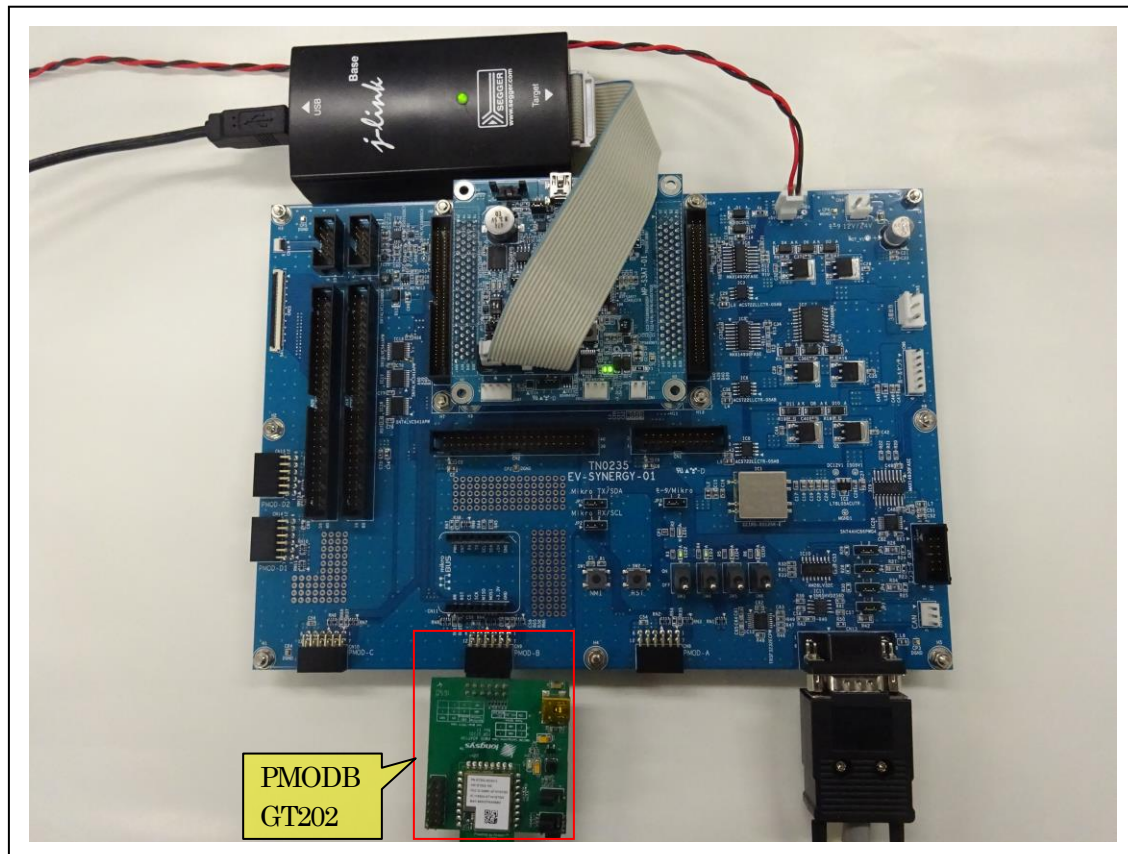
【WiFi_DHCP_TCP_GT202_PMODB】
